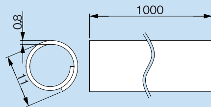
寸法図
