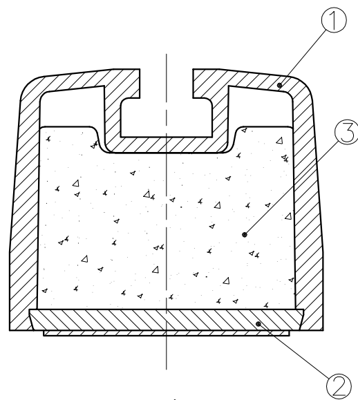
X-X'断面
