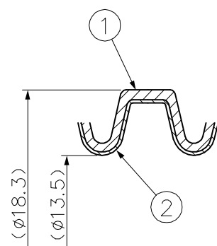
Ⓐ 部詳細 (SCALE: 5/1)
