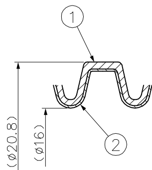
Ⓐ部詳細 (SCALE: 5/1)
