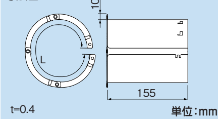
寸法図
