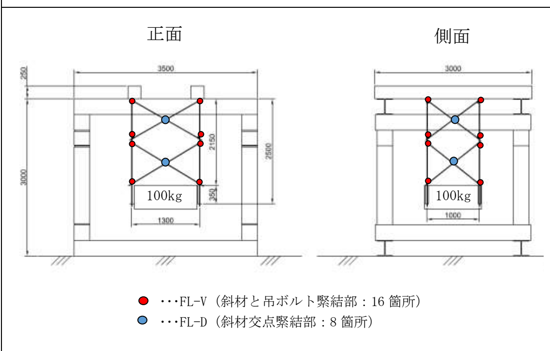
試験体の構造及び寸法図
