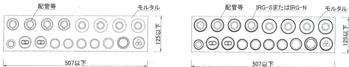
正面図
