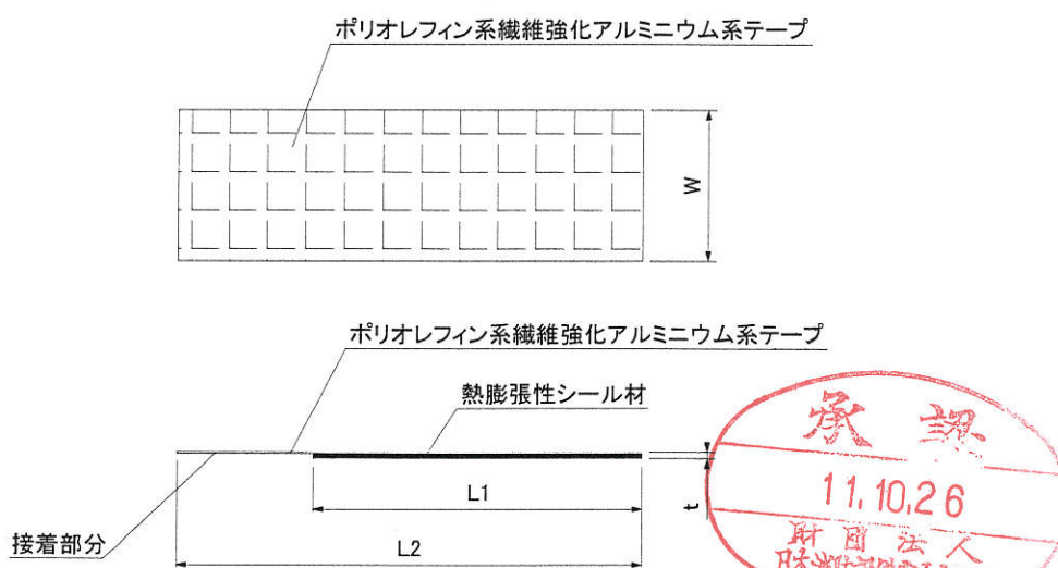
図2 構造
