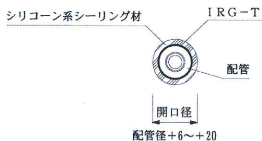
正面図
