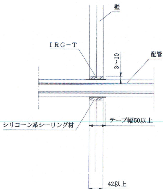
断面図
