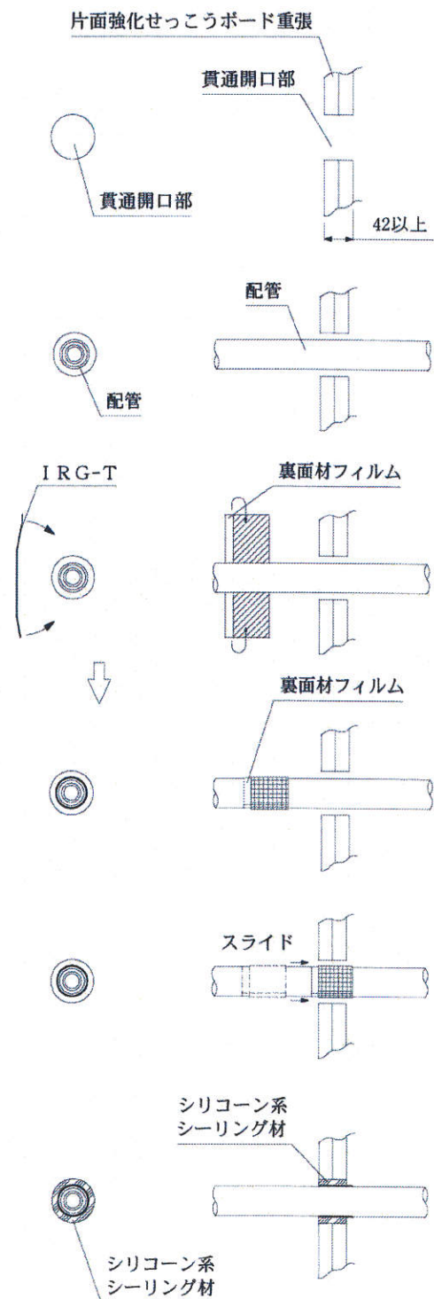
<正面図>
