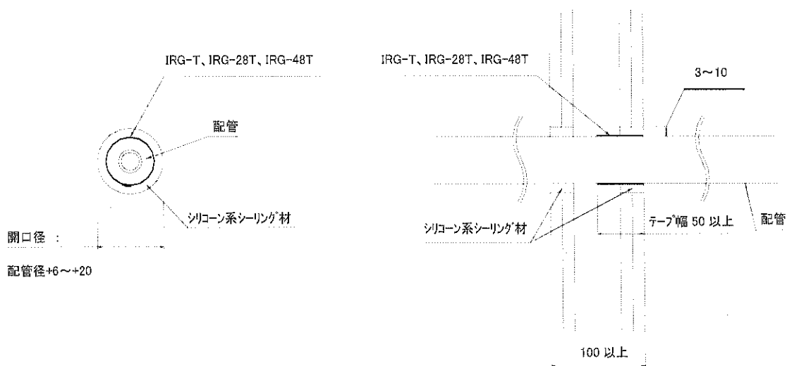
施工断面図
