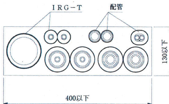
正面図
