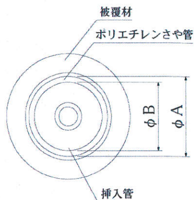
挿入管②
