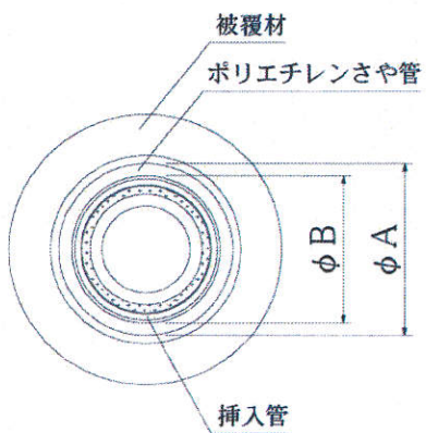
挿入管③
