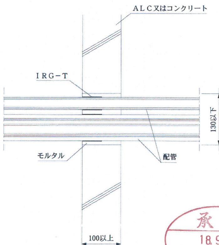
断面図
