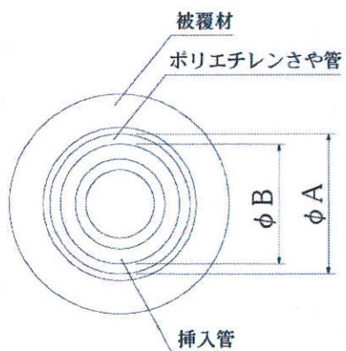
挿入管①
