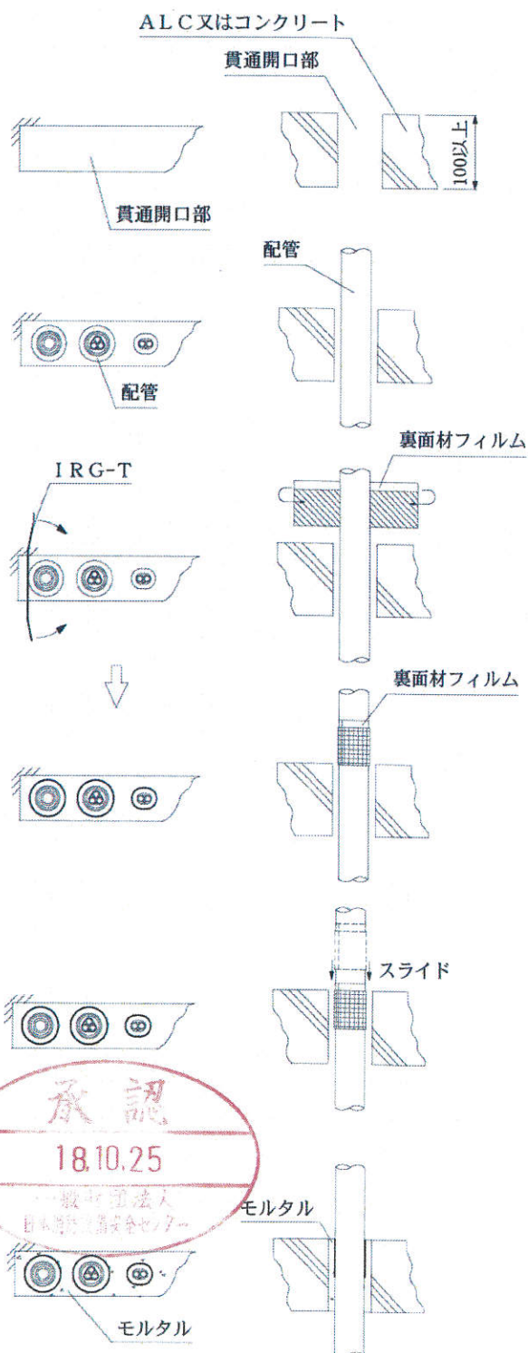
<側断面図>
