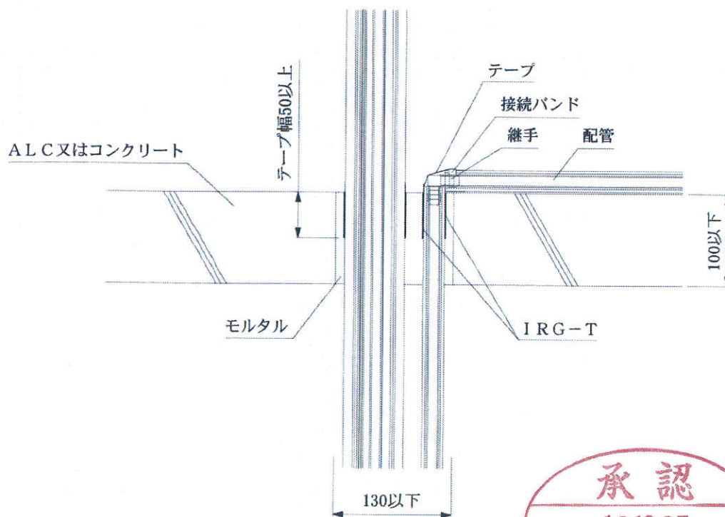
断面図
