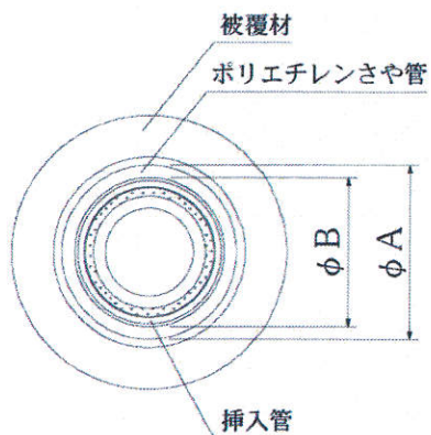
挿入管③
