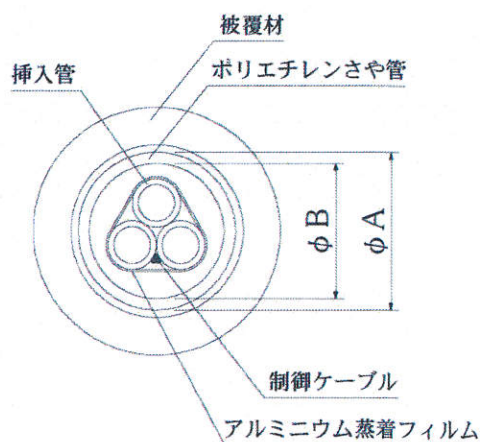
挿入管④、⑤
