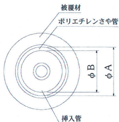
挿入管②
