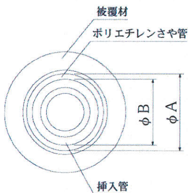
挿入管①
