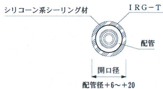
正面図
