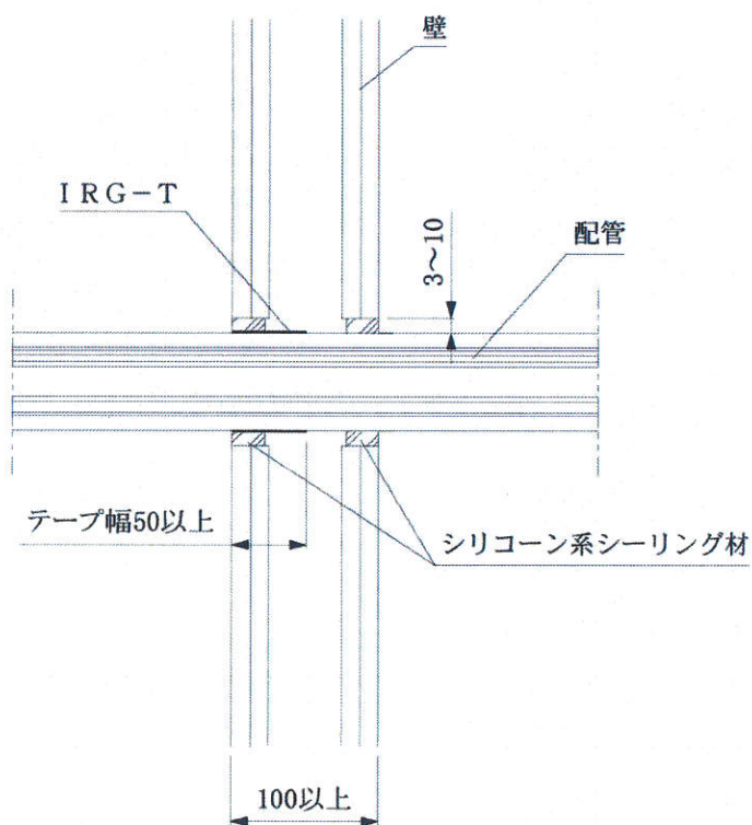
断面図
