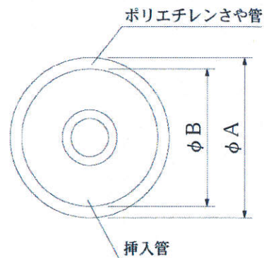
挿入管②
