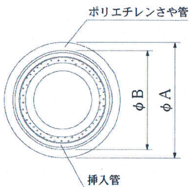
挿入管①
