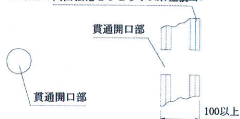
<正面図 断面強化せつこう糸側断面図>
