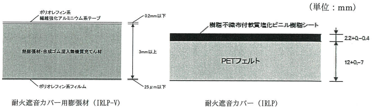
図1 断面図
