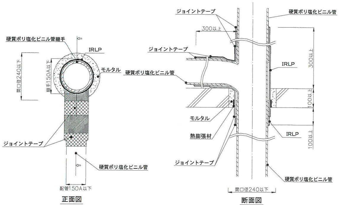
継手図
