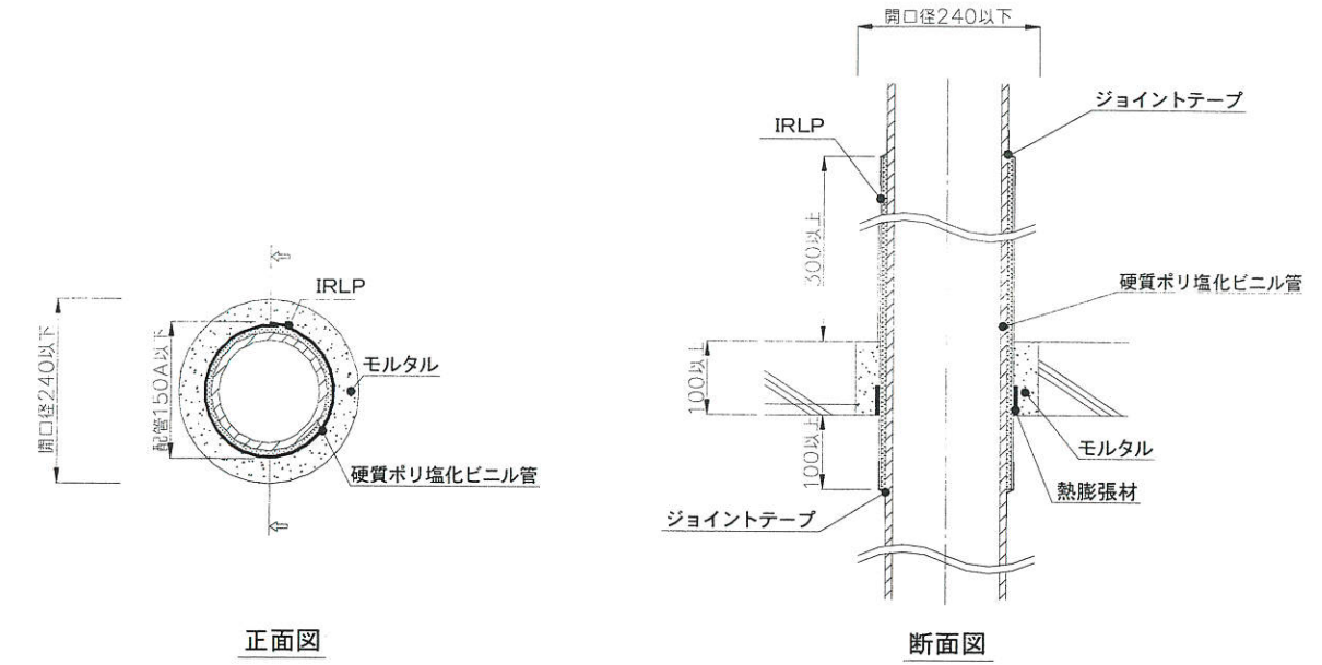
直管図
