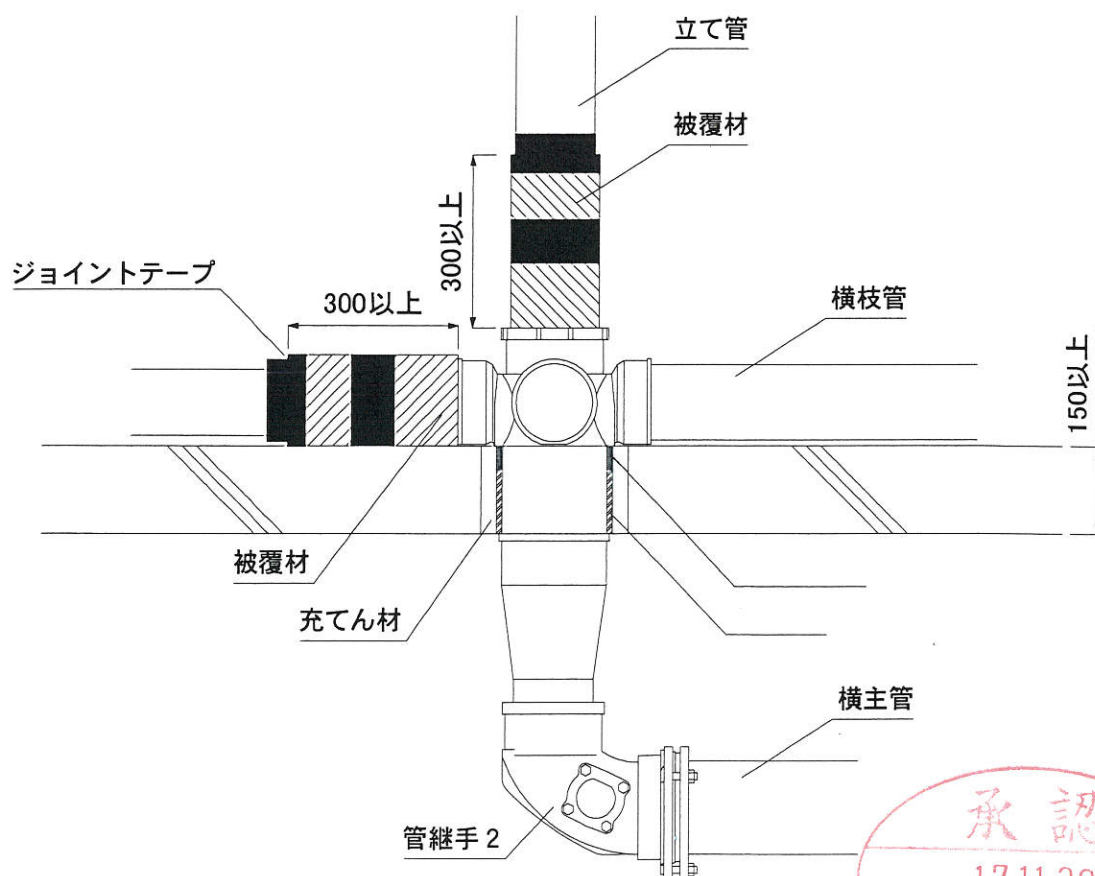
図2 断面図
