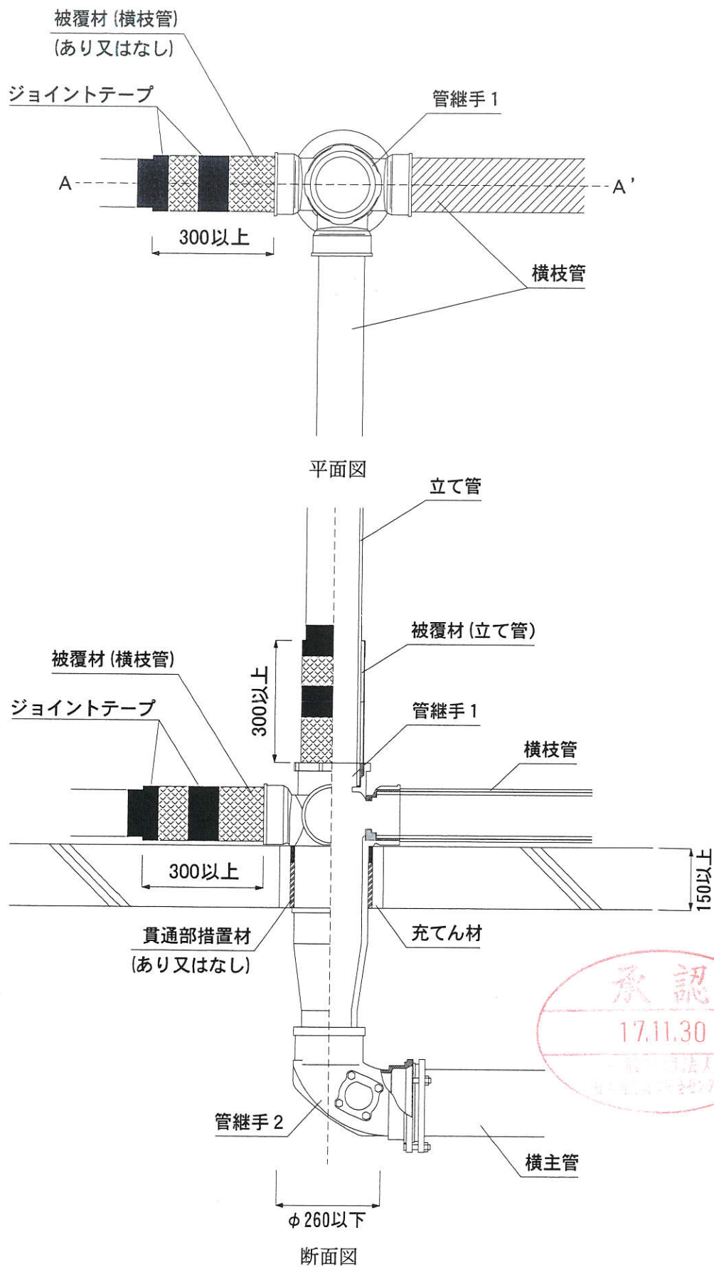
図 4 標準施工図
