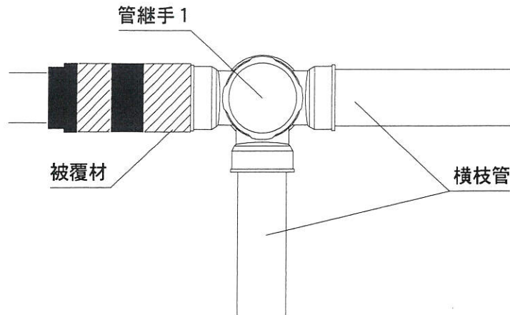
図1 平面図
