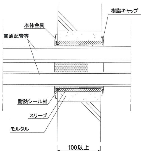
図-1 I R M-Nを貫通配管に施工した構造
