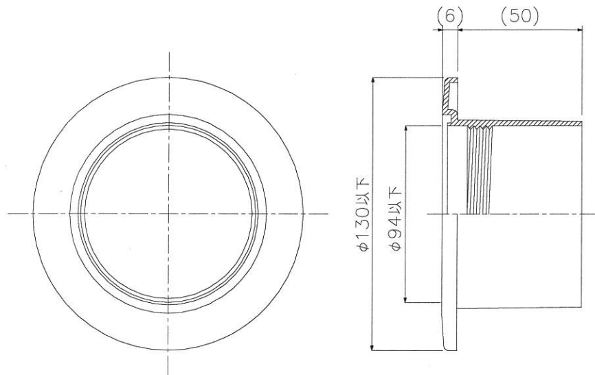
図－3 樹脂キャップの形状
