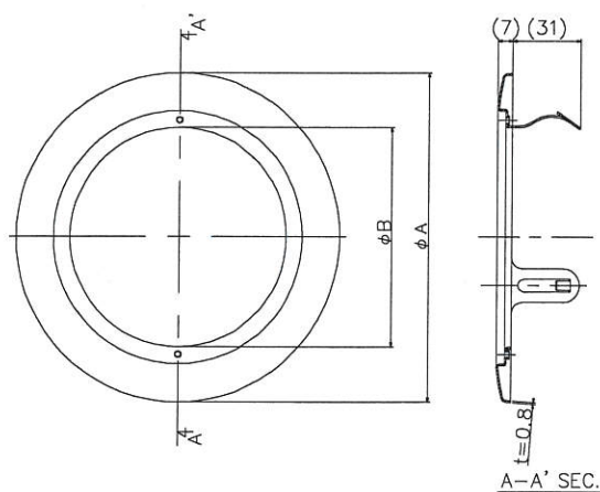
図－2 IRM-N（耐火キャップマンションタイプN）の形状
