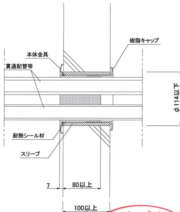
断面図
