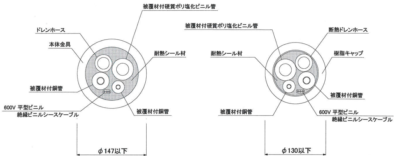
正面図(金具側)
