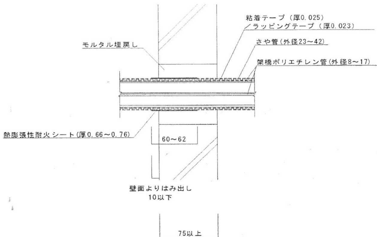
<断面図>
