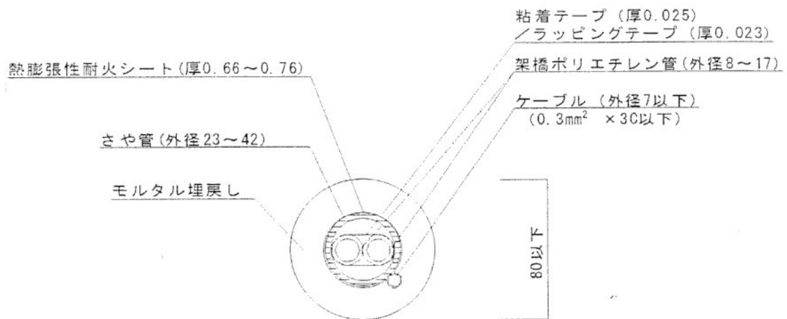
<正面図>
