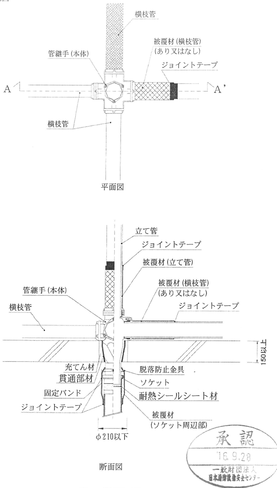
図5 標準施工図
