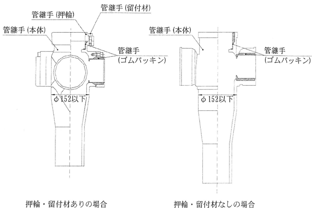
図4 管継手詳細図 (代表例)
