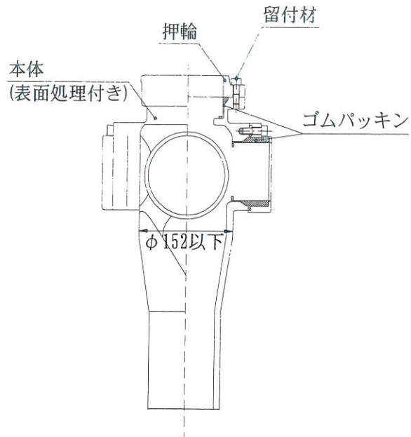
図3 管継手詳細図（代表例）
