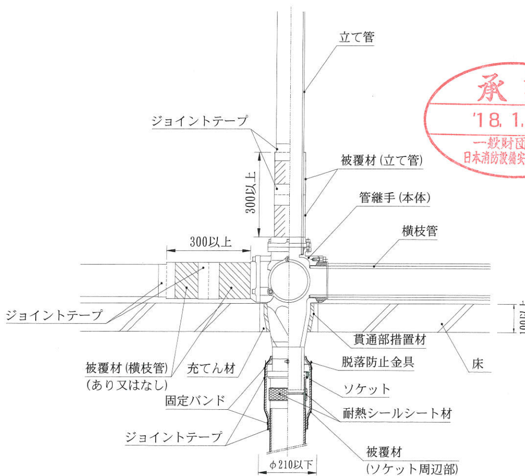
図2 断面図
