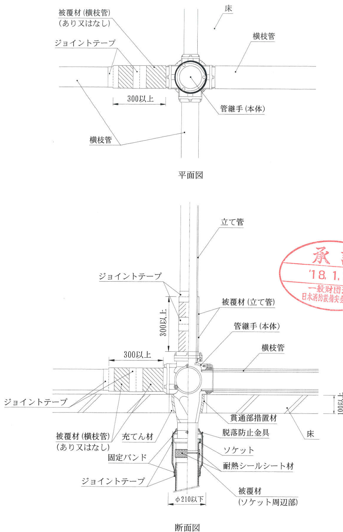
図4 標準施工図
