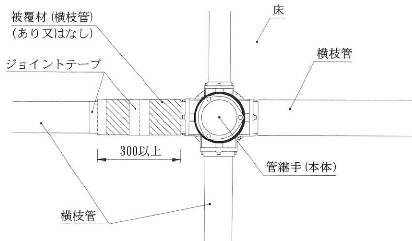
図1 平面図
