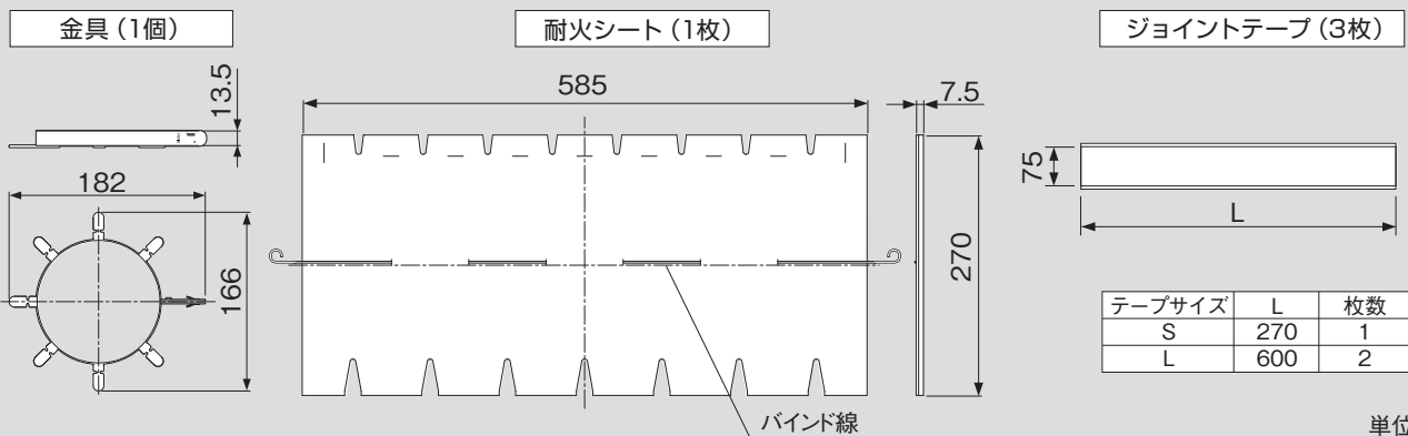
金具付耐火シート (IRXP-SK-B)
