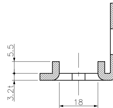
X-X' 断面图
