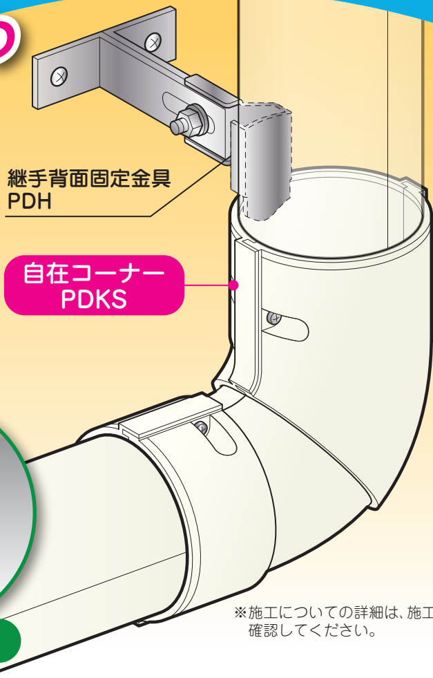
ひねり施工
