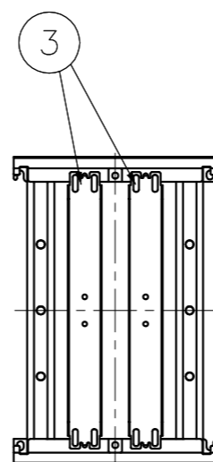
フタ補強板取付け位置
