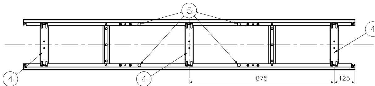
フタ補強板・樹脂ブッシュ取付位置
