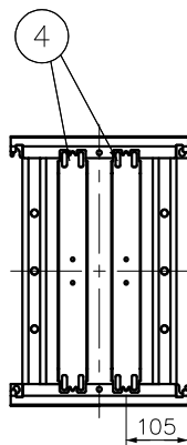
フタ補強板取付け位置
