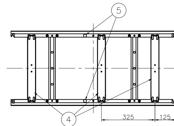
フタ補強板・樹脂プッシュ取付位置
