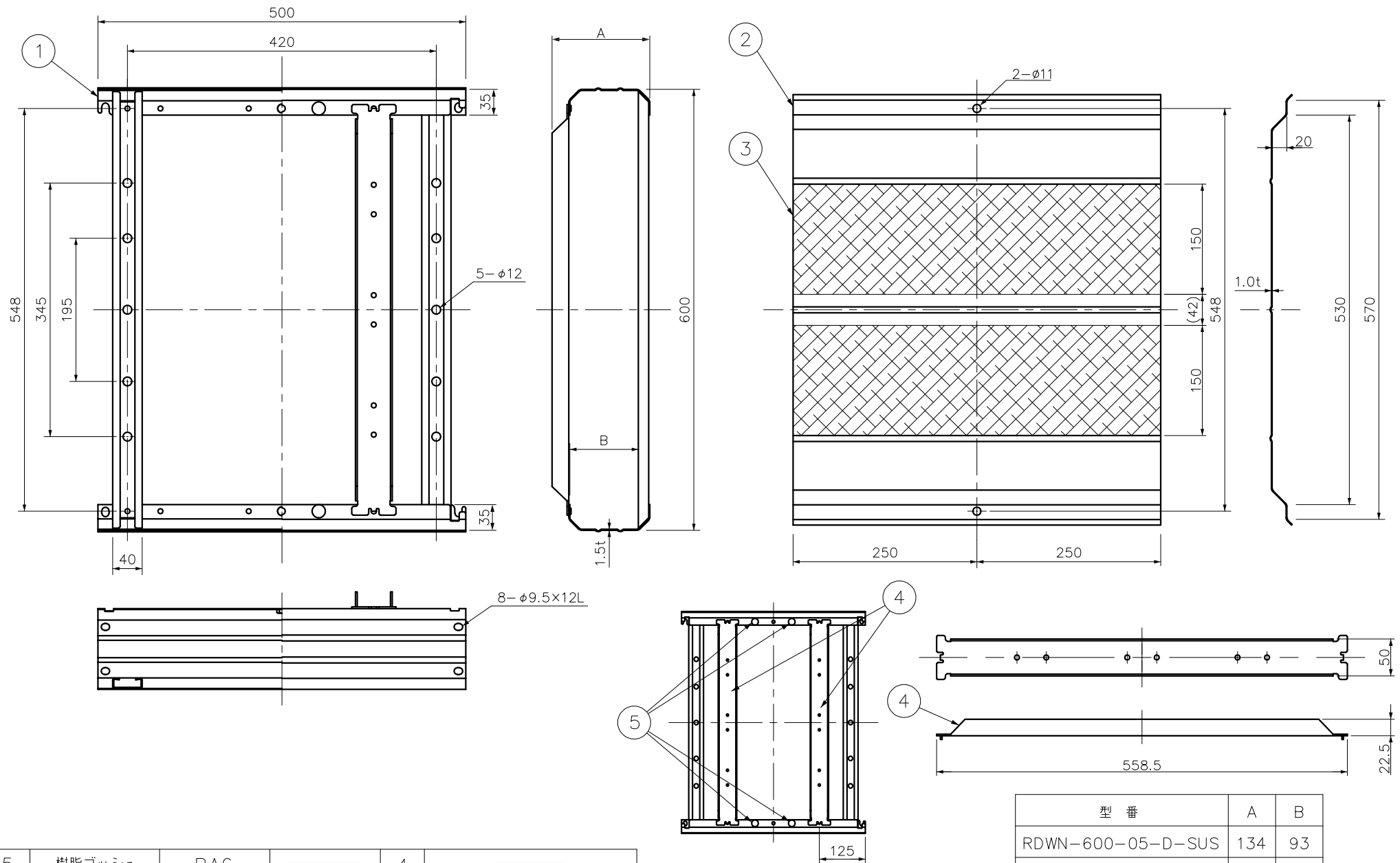
フタ補強板・樹脂ブッシュ 取付位置
