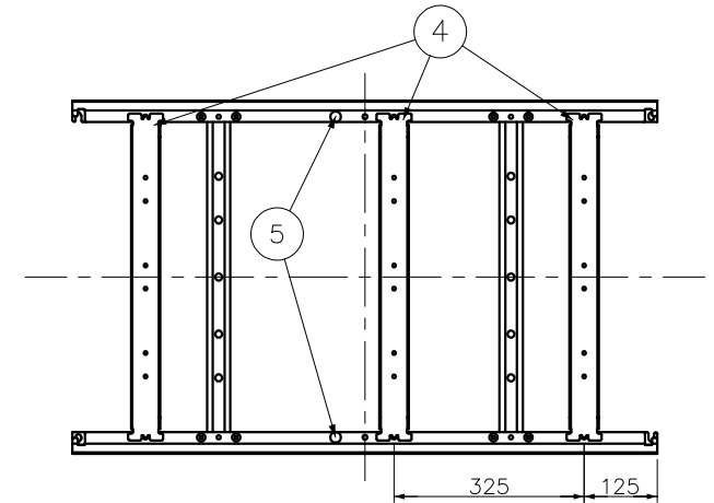
フタ補強板・樹脂プッシュ取付位置
