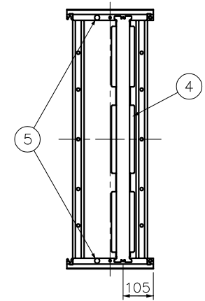
フタ補強板・樹脂プッシュ取付位置
