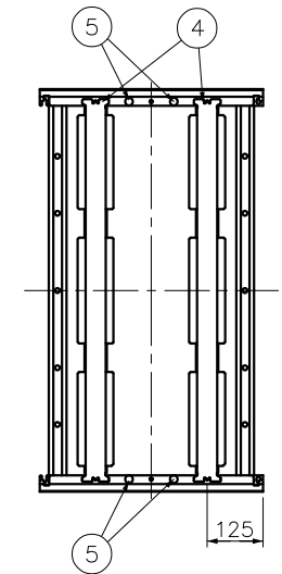
フタ補強板・樹脂ブッシュ取付位置
