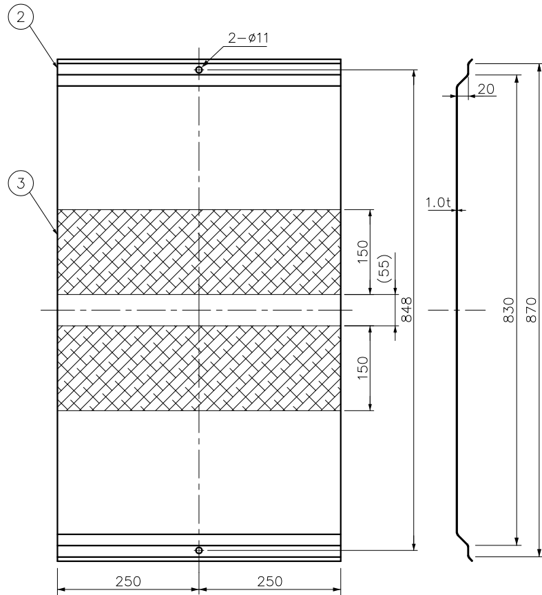
フタ補強板・樹脂ブッシュ取付位置
