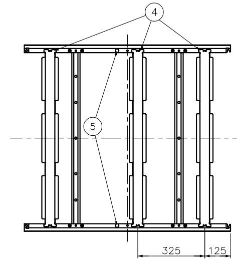
フタ補強板・樹脂プッシュ取付位置
