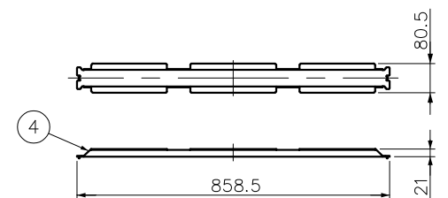
フタ補強板・樹脂ブッシュ取付位置
