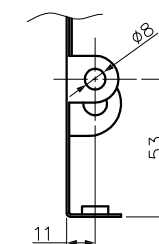
A矢視図
