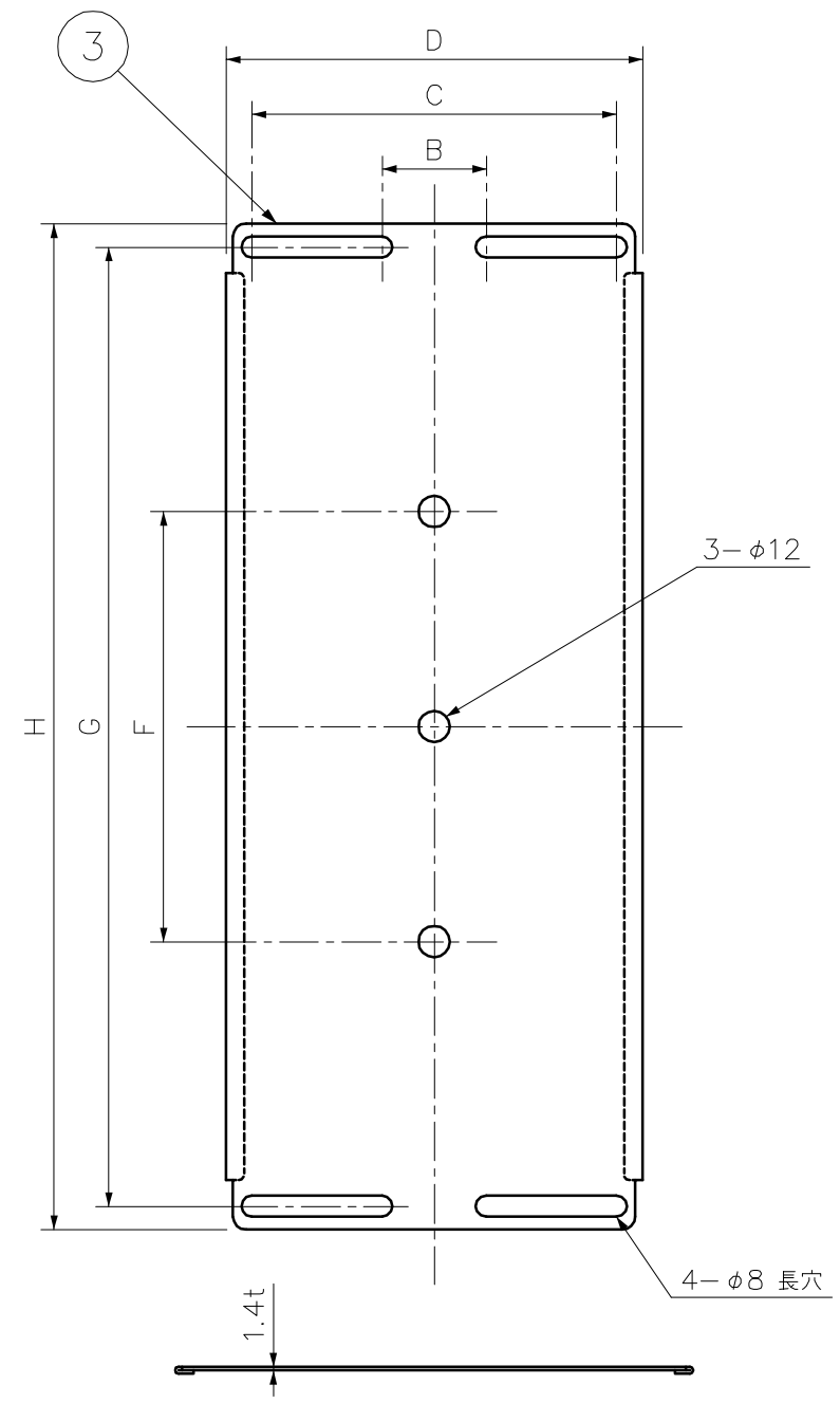
底 板
