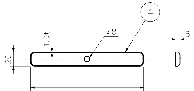
当 て 板
