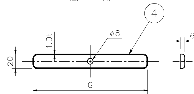
当 て 板
