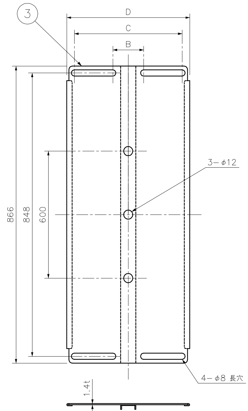
底 板
