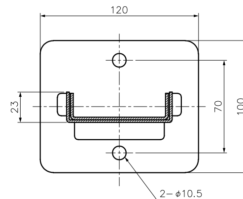
A-A' 断面図
