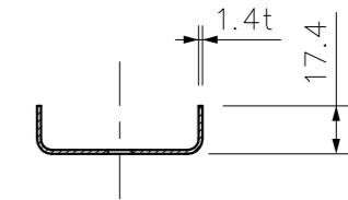
A-A' 断面図
