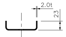
A-A' 断面図
