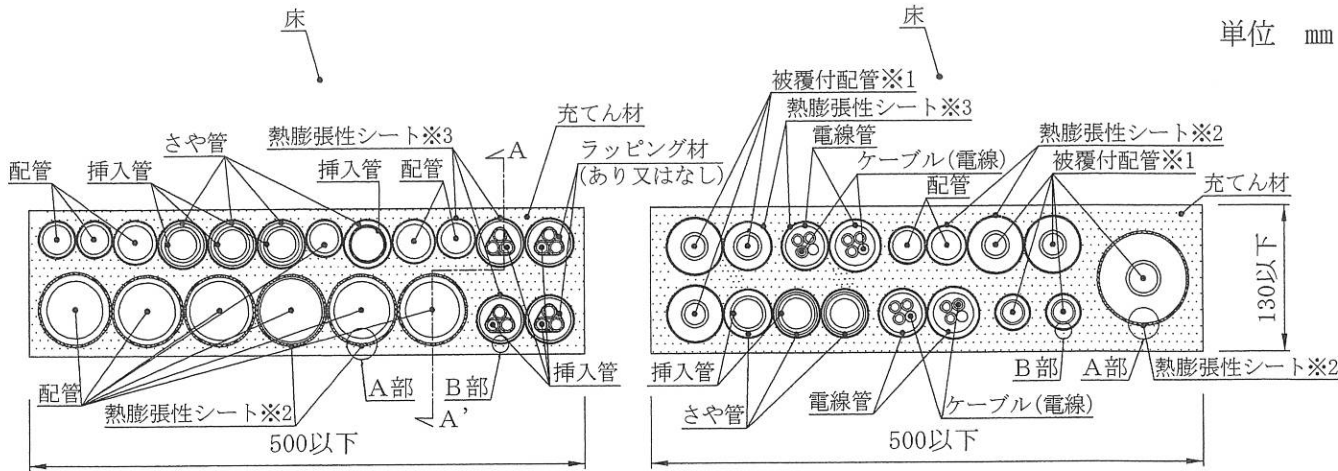
平面図 ケーブル・配管等の配置(例1) 平面図 ケーブル・配管等の配置(例2)
