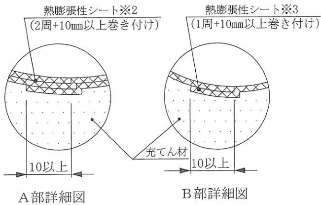
熱膨張シートの重なり代部詳細 注) ケーブル・電線管・さや管・配管・挿入管の配置の一例を示す ※1) 被覆材(あり又はなし) ※2) 熱膨張性シートが2周+10mm以上巻き付けの場合 ※3) 熱膨張性シートが1周+10mm以上巻き付けの場合
