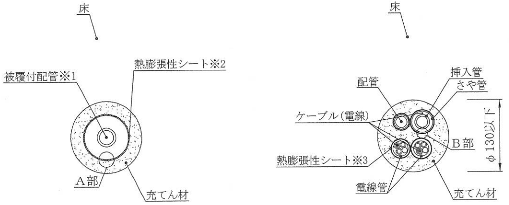
平面図 ケーブル・配管等の配置(例1) 平面図 ケーブル・配管等の配置(例2)
