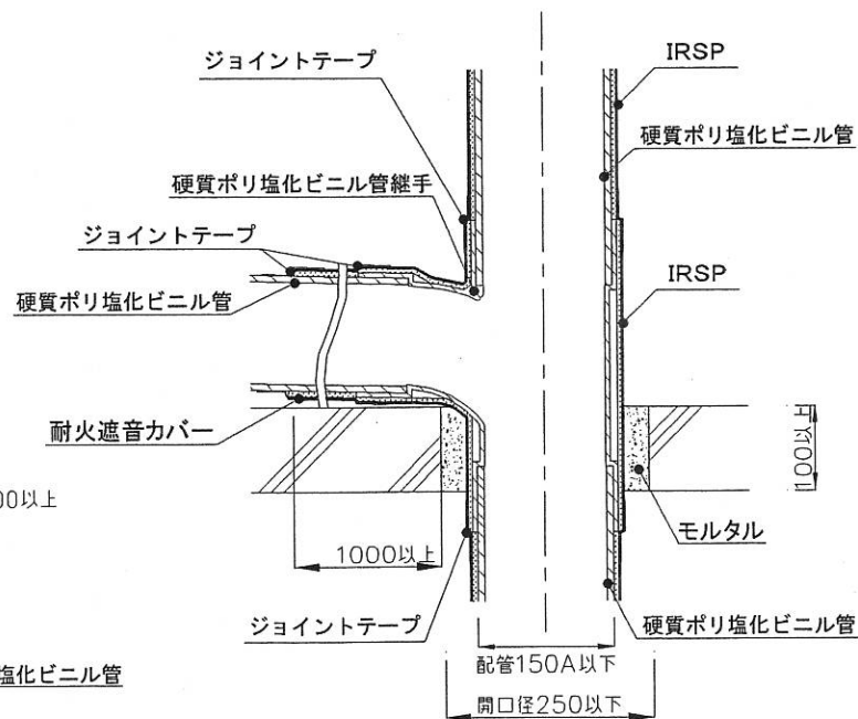
断面図
