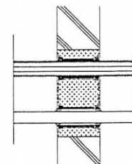
施工図（手順）
