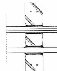
施工図 (手順)
