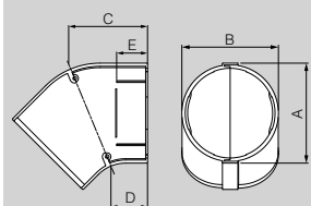
Dimensions
