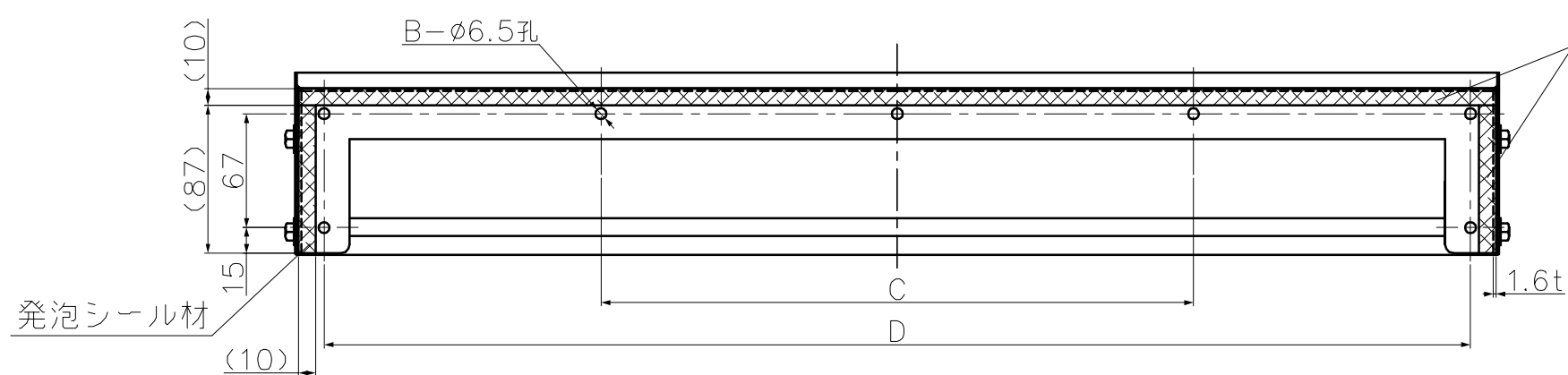
《背面図》
