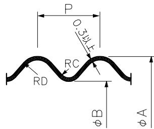
Y 部 詳 細
