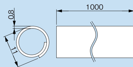
寸法図
