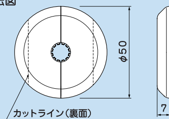
寸法図
