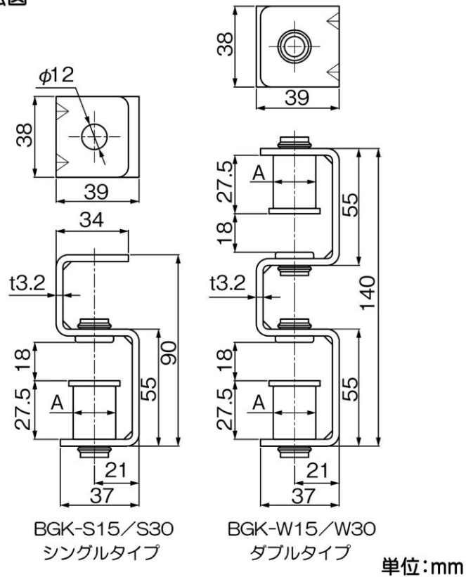
寸法図
