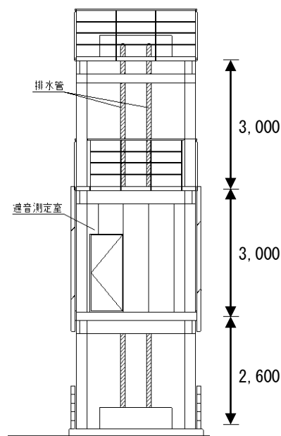
図 1. 排水タワー
