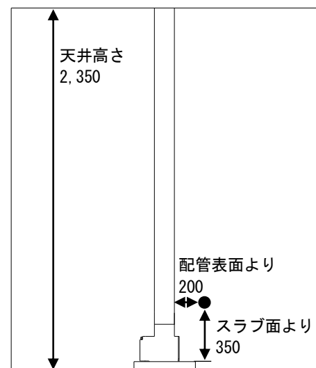
図 2. 測定室内及び騒音測定位置
