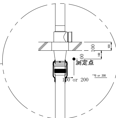
図 4. 測定室内及び騒音測定位
