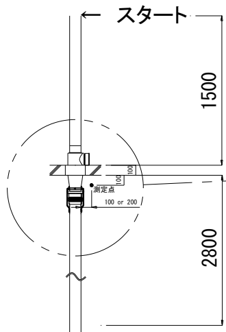
図 3. 排水経路図
