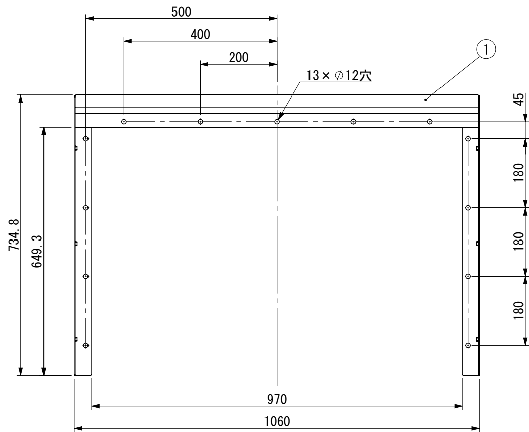
フレーム寸法詳細図
