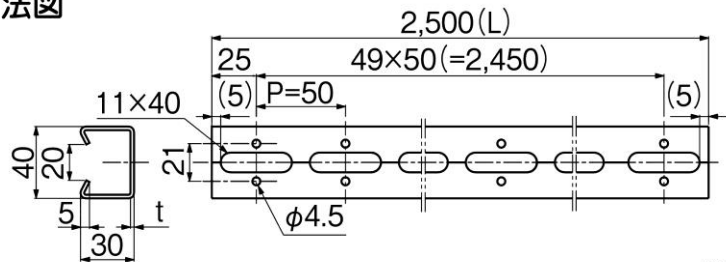
寸法図
