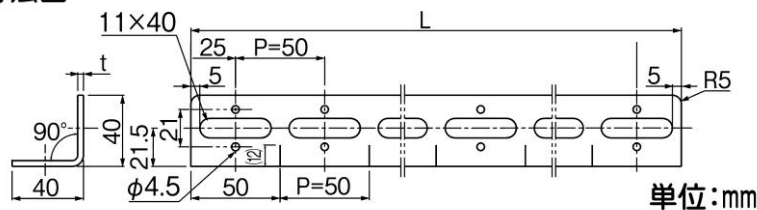
寸法図
