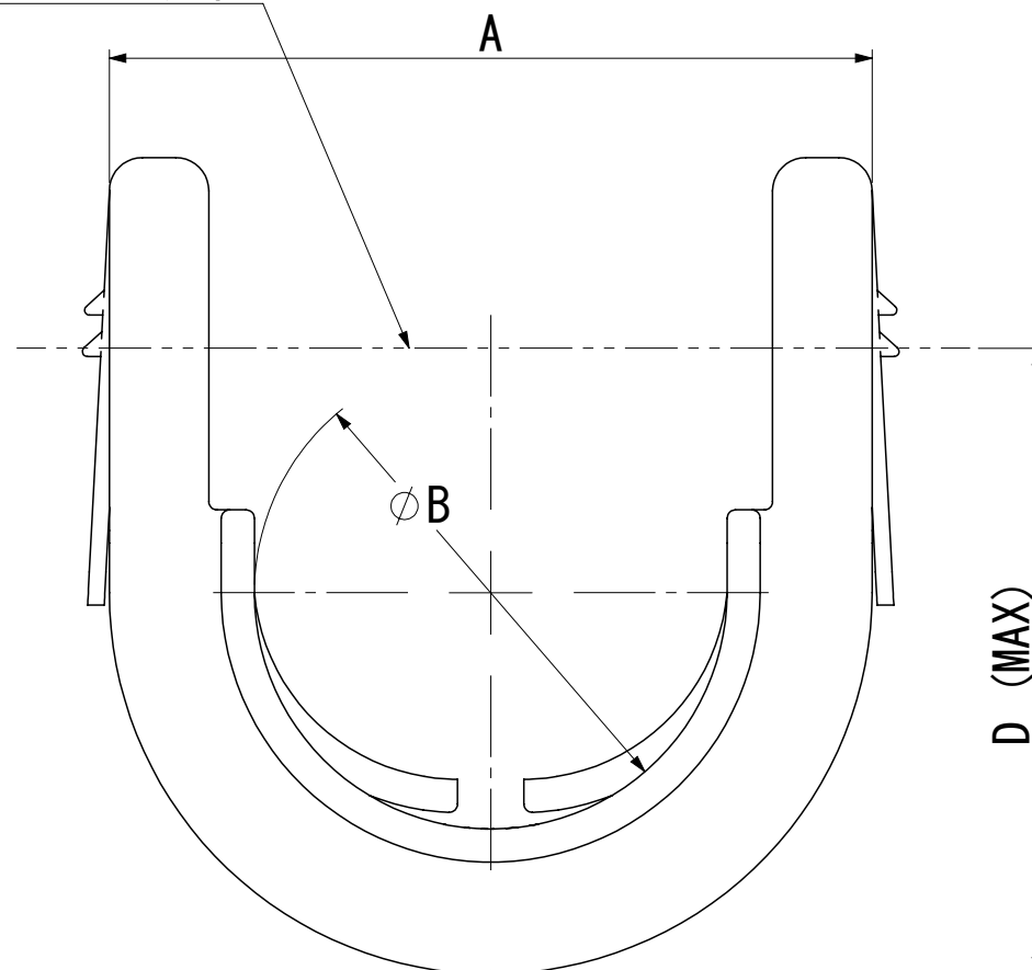
取付ベース (CSB-BL/BH) サドル差込面
