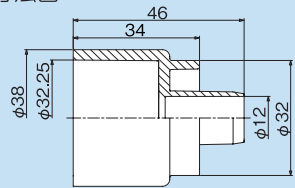
寸法図
